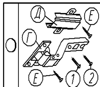
Крепление стяжки эксцентриковой (комплект №45)
