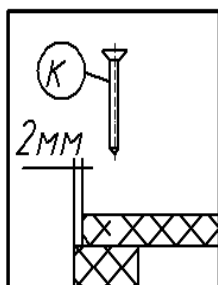
Крепление задней стенки (комплект №10)
